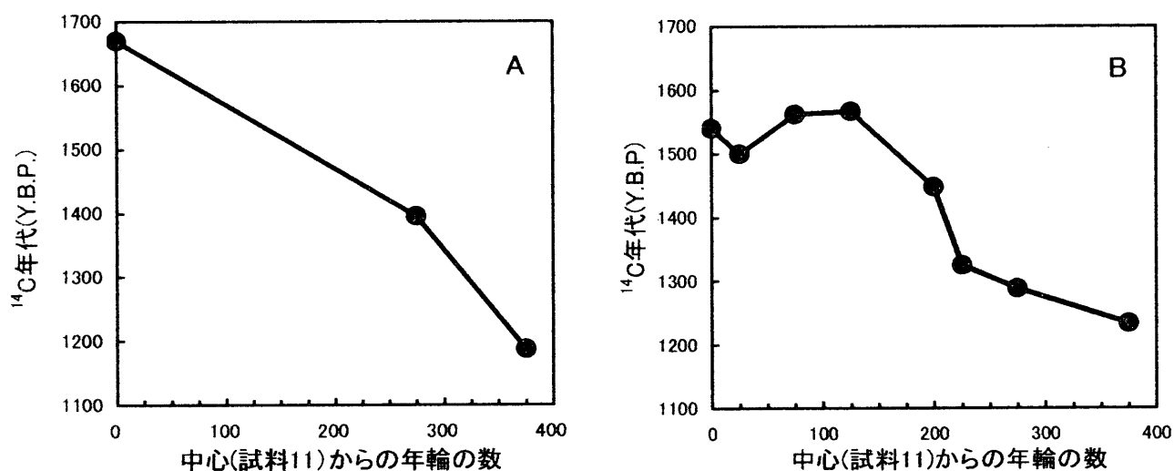
図 1 年輪数と ^{14}\text{C} 年代の関係 (A: 測定(a), B: 測定(b))
